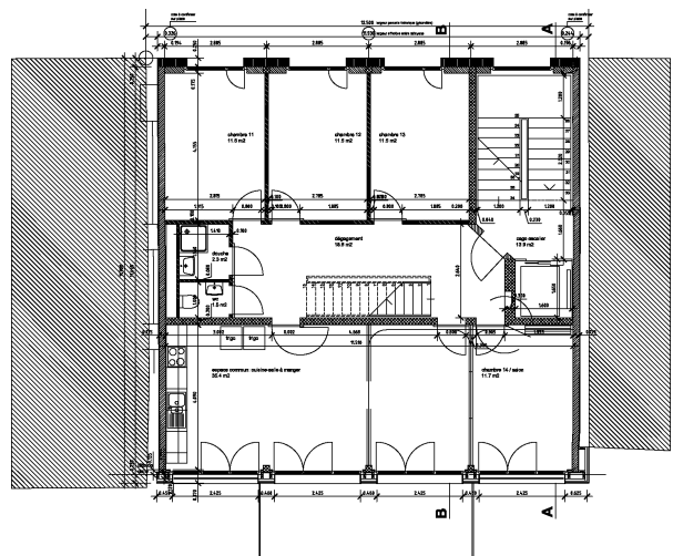
Plan de l'étage-type
